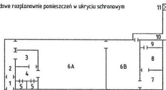
Przykładowe rozplanowanie pomieszczeń w ukryciu schronowym
